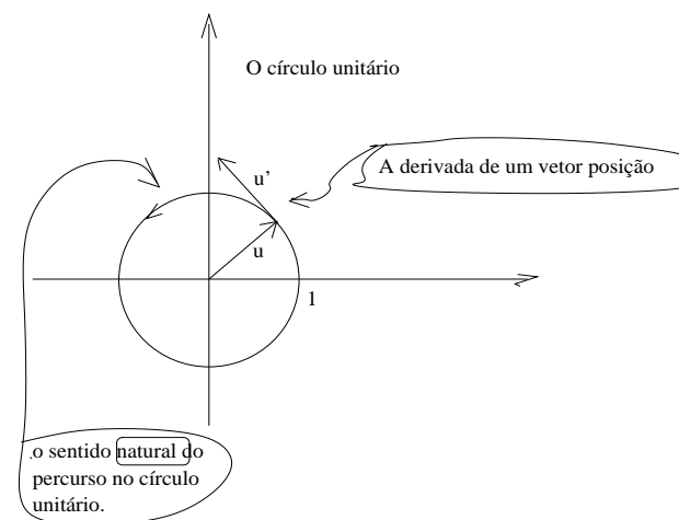
Figura 1: O círculo unitário
